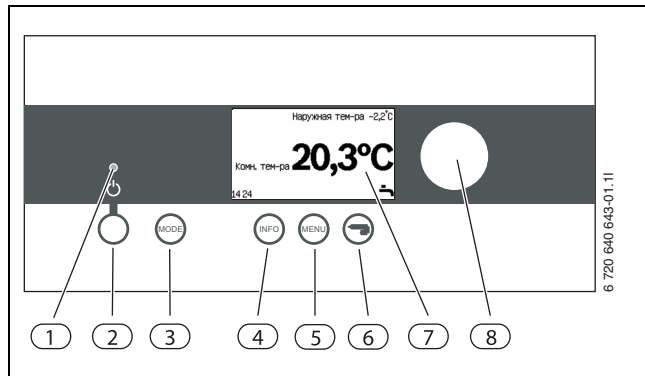
Рис 3 Панель управления
